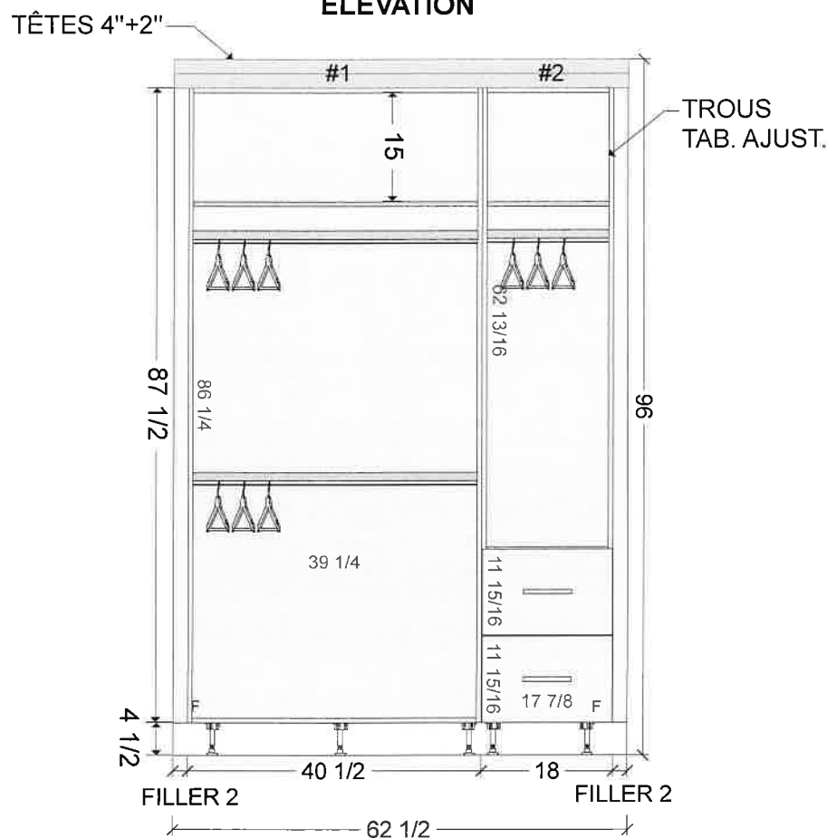
CHAMBRE D'INVITÉS - ÉLEVATION
